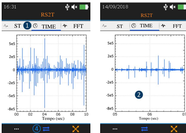
Figura 14-1: ingrandimento e restringimento della forma d'onda temporale
