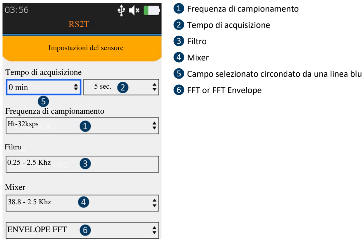
Figura 10-2 Impostazioni della misurazione ad ultrasuoni
