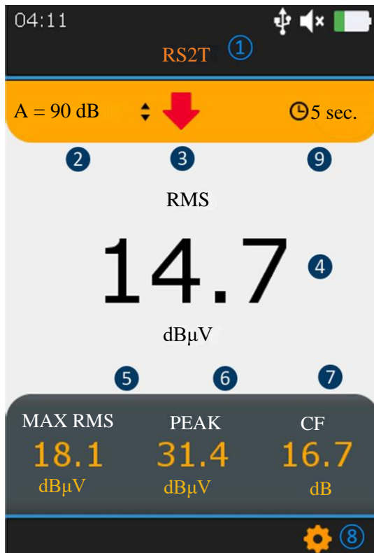
Figura 10-1 Schermata di misurazione ad ultrasuoni
