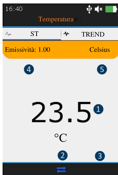
Figura 16-1: Schermata della temperatura di corrente
