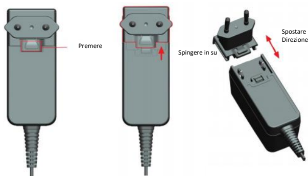
Figura 6-2 Sostituzione della spina principale dell'alimentatore
